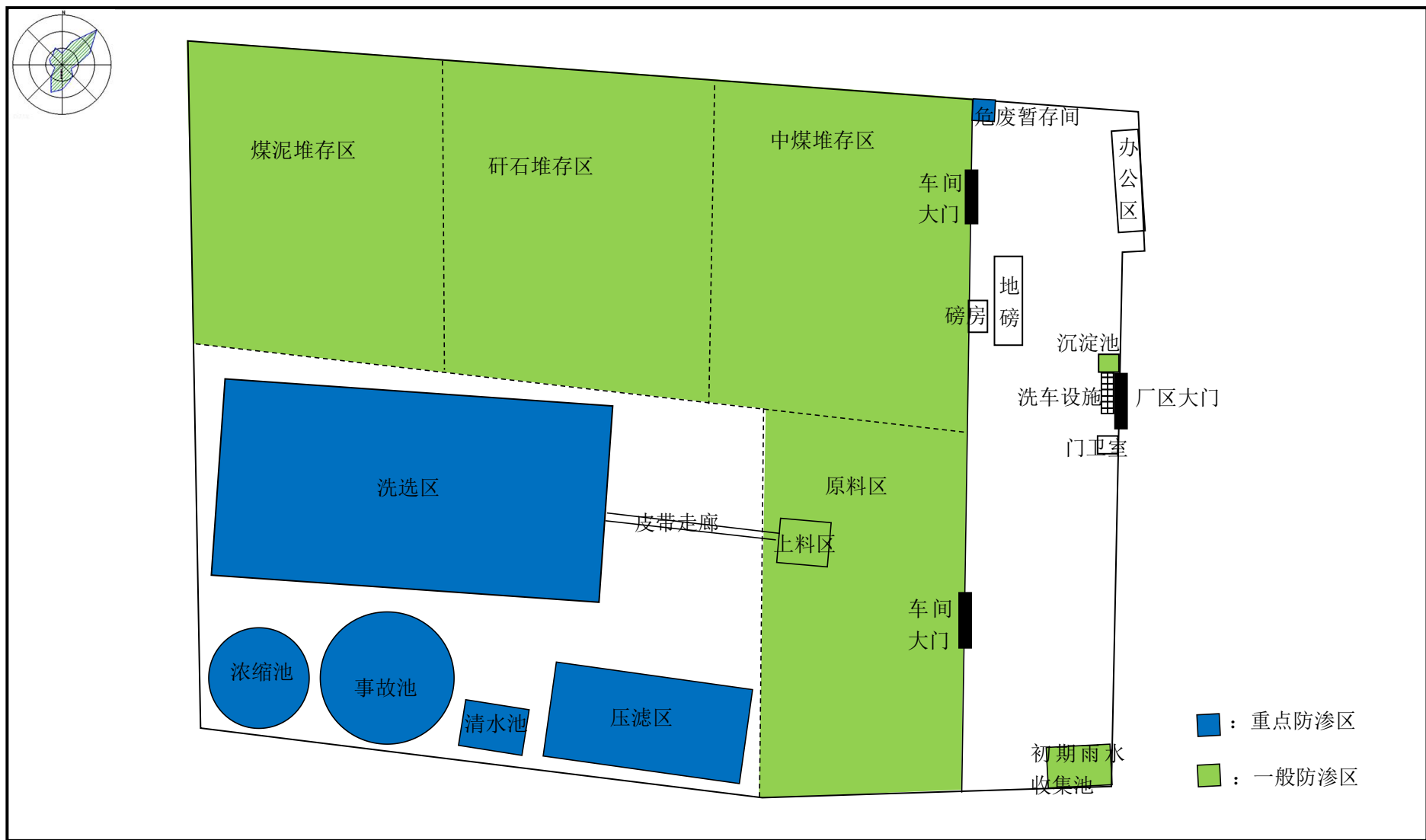
附图4 本项目厂区平面布置示意图
