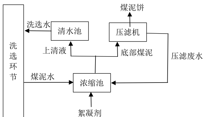
图2-5 项目煤矸石洗选废水处理工艺流程示意图
